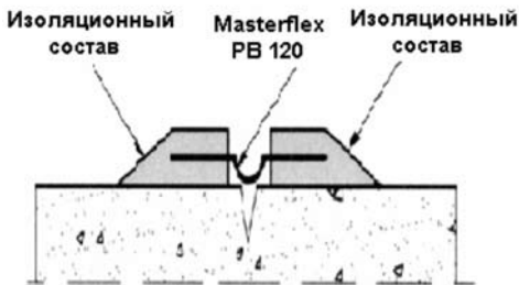
Рис 2. Изоляция трещин
